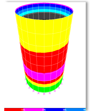
Analisi FEM Steel stack
